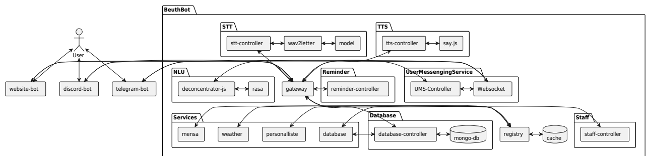
BOT-16: Support mehrerer Messenger-Typen durch Umbau der Benutzererkennung
